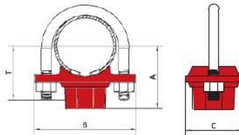
Рис.1. Габаритные размеры отвода (седелка) Ubolt «LEDE».
