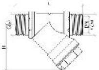
Фильтр сетчатый муфтовый косой с краном для промывки, 4004 Aquasfera
