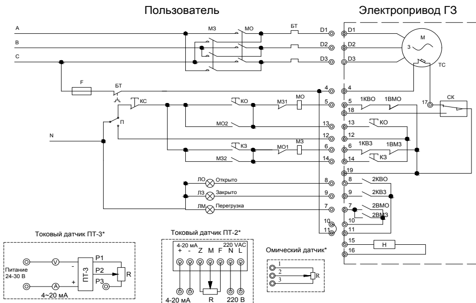
Рис. 6(1) Электрическая схема управления для электроприводов серии ГЗ-А и ГЗ-Б.
