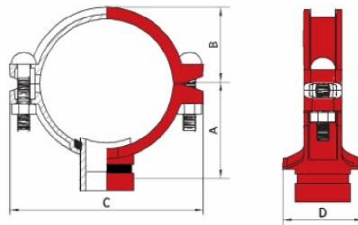
Рис.1. Габаритные размеры отвода (седелка) под муфту «LEDE».
