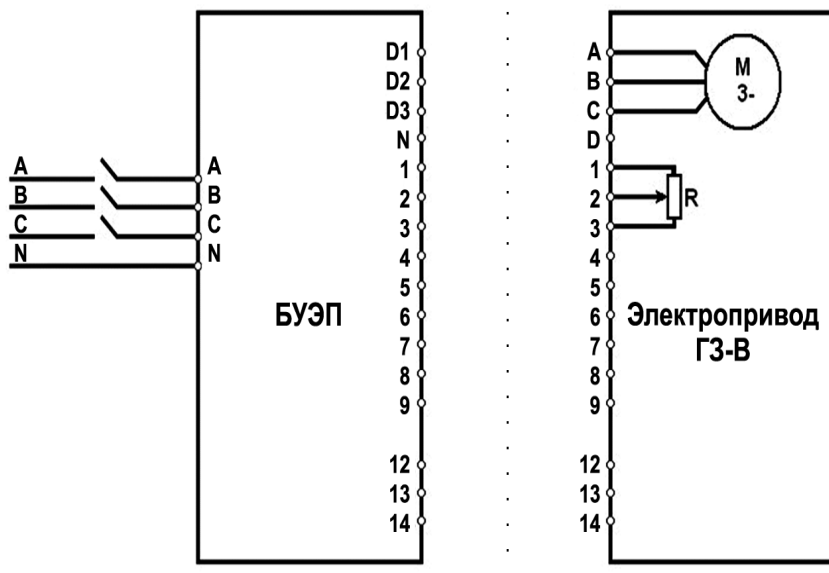
Рис. 7 Блок-схема подключения БУЭП к электроприводу
